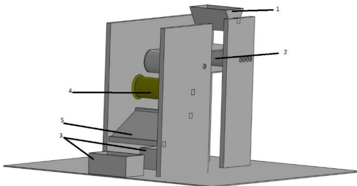
Рис. 1. 3D-модель производственной линии: 1 – бункер подачи отходов; 2 – конвейер; 3 – бункеры приема отходов; 4 – магнитный сепаратор; 5 – скат
