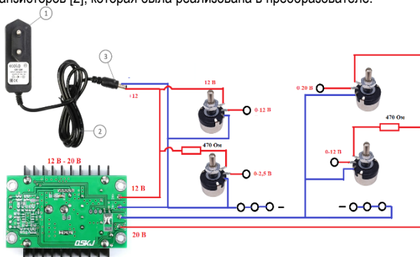
Рис. 3. Разработанная принципиальная схема макета
