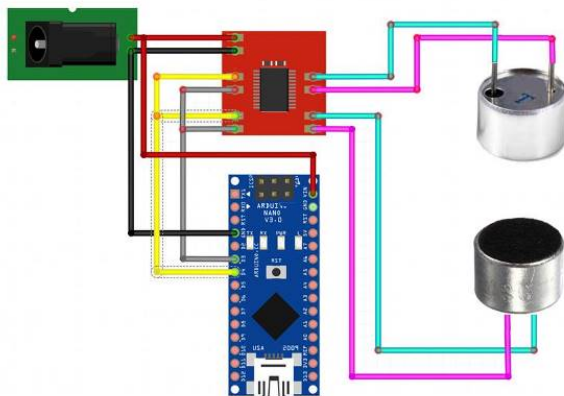
Рис. 7. Схема подключения
