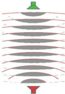
Рис. 1. Метод «Стоячая волна»
