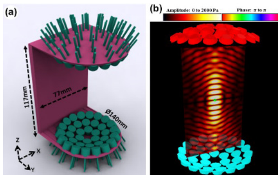
Рис. 6. Трехмерное удержание и движение частиц: а) – визуализация модели ультразвукового излучателя на основе эффекта стоячей волны; б) – срез амплитудного поля с частицей, помещенной в один из узлов, цвет преобразователей представляет их фазу излучения
