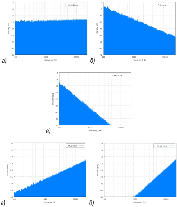
Рис. 2. Амплитудно-частотная характеристика (АЧХ) разных видов шумов: а) белый шум; б) розовый шум; в) красный шум; г) синий шум; д) фиолетовый шум
