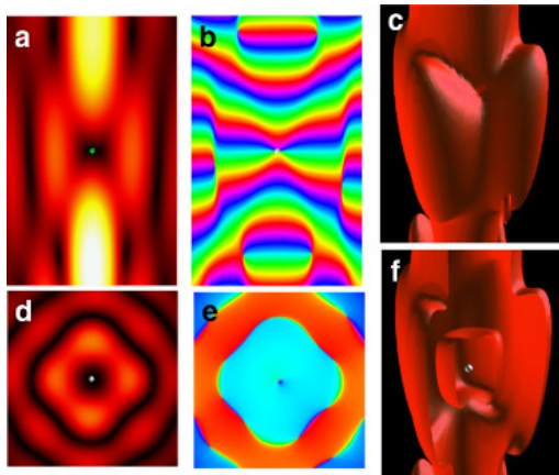
Рис. 5. Бутылочные акустические ловушки Bottle trap
