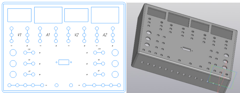
Рис. 2. Внешний вид и модель разрабатываемого макета
