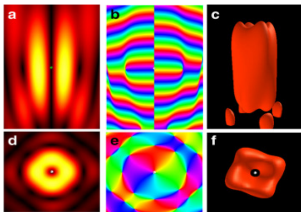
Рис. 4. Вихревые акустические ловушки Vortex trap
