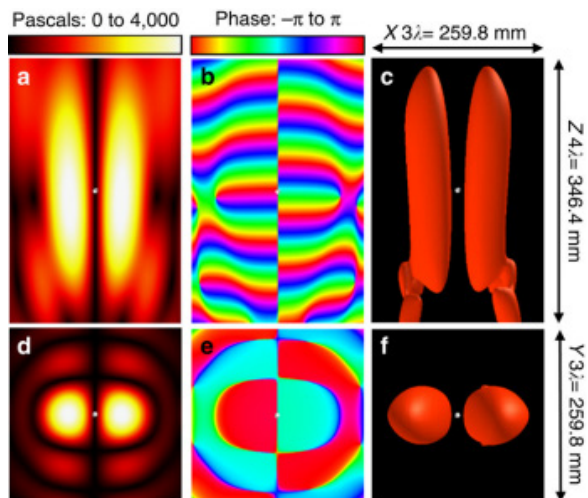
Рис. 3. Двойные акустические ловушки Twin trap
