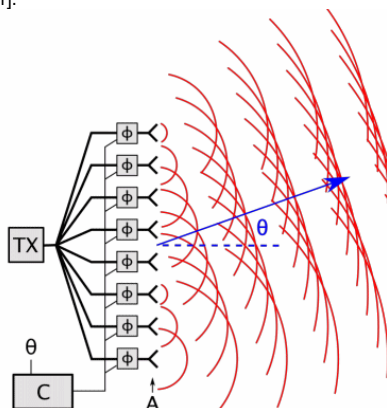
Рис. 2. Метод «Фазированные решетки»
