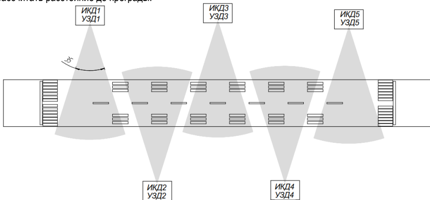
Рис. 3. Схема расположения инфракрасных (ИКД) и ультразвуковых датчиков (УЗД)
